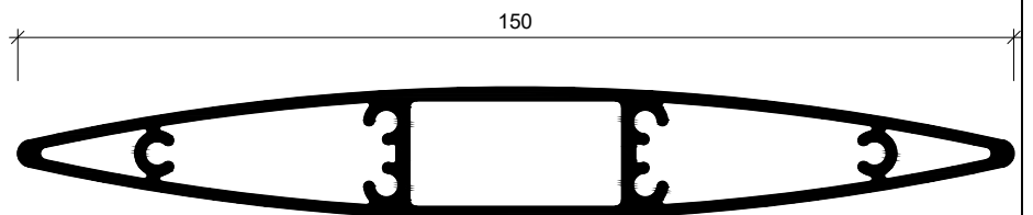
MF150 BLADE
