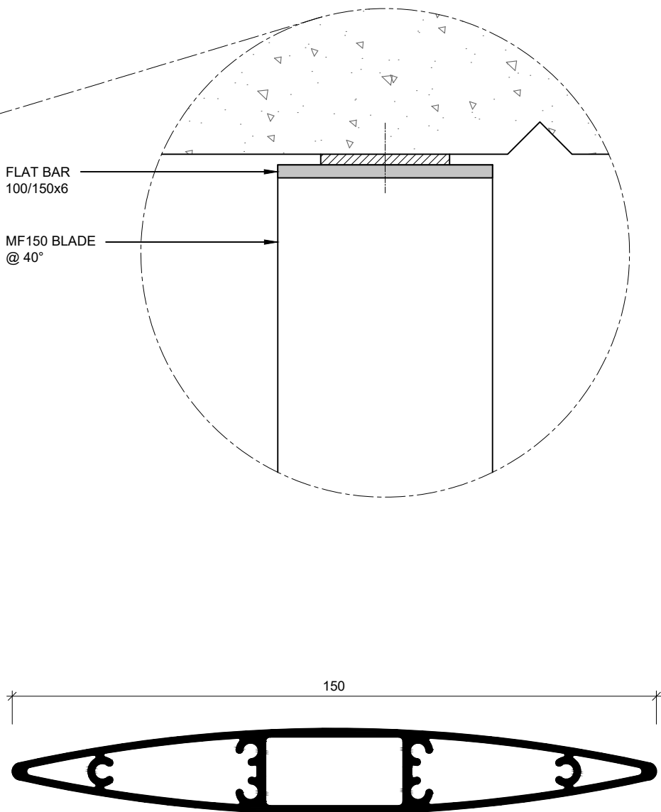
MF150 BLADE
