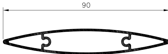
MS90 BLADE
